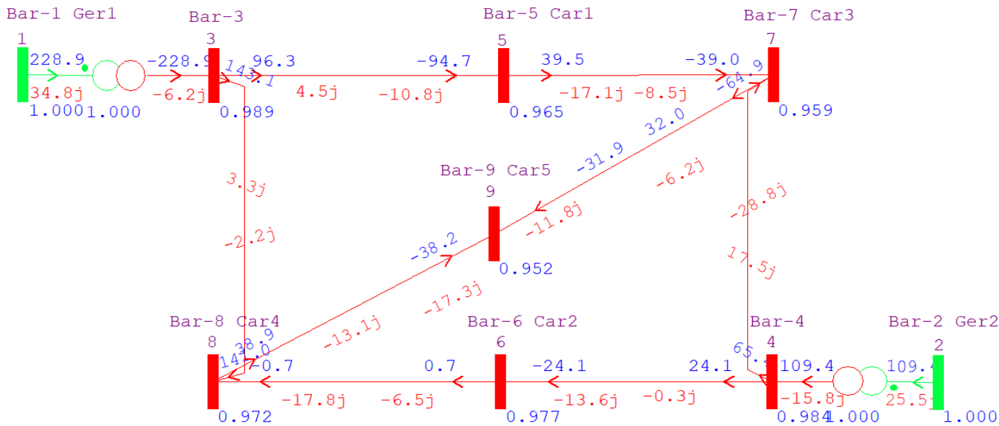
Diagrama no ANAREDE do STB-9 – Caso base
