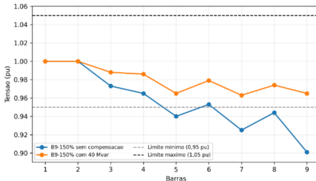
Comparação das tensões na barra antes e depois da compensação
