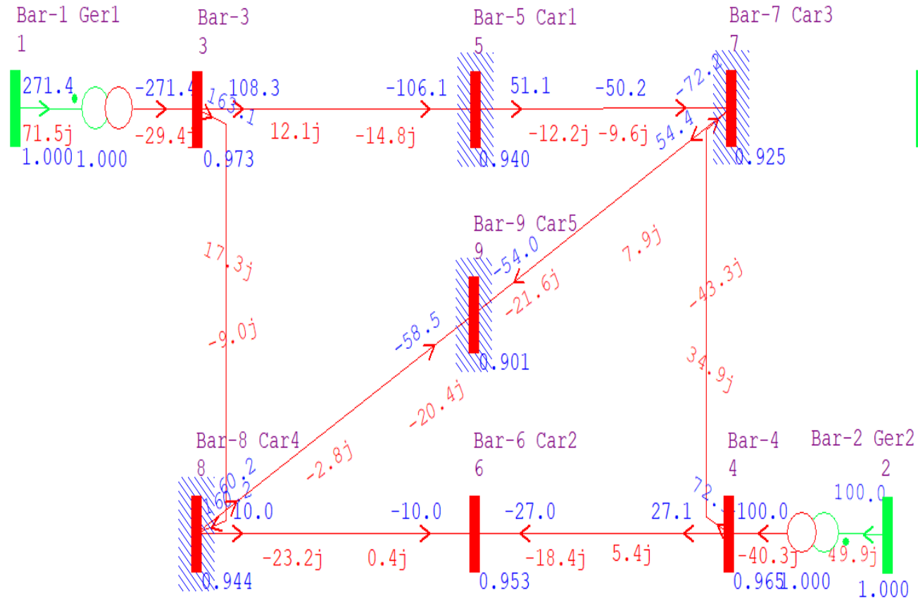
Diagrama no ANAREDE do STB-9 150% na barra 9 sem compensação
